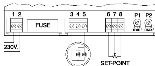
Fig. D SCHEMA COLLEGAMENTI
